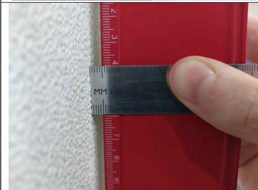
Фото №11. Измерения уровня стен в прихожей.
